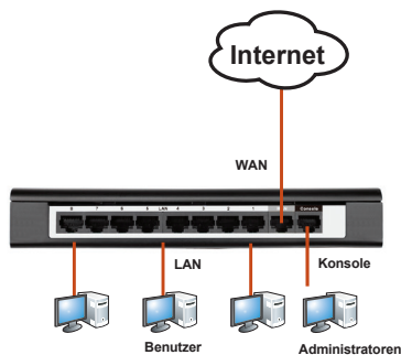
Abbildung 4: Einfaches Verkabelungsbeispiel
